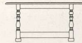
テーブル K-683 W140 × D85 × H65 (甲板ムク材)
