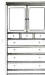
チェストオブドロワー K-608 W105×D47×H180
